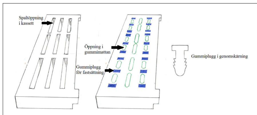
Figur 2. Betongspaltelement till vänster och till höger illustreras samma element med en gummimatta ovanpå
